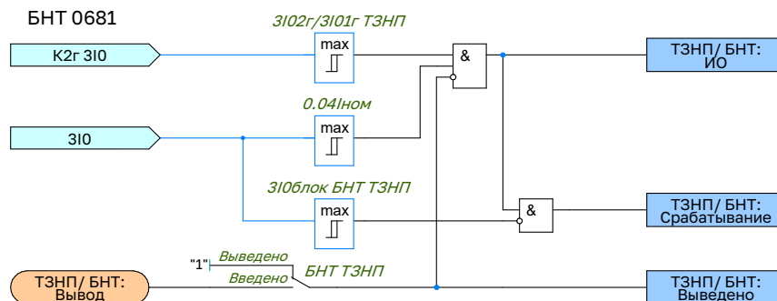
Рисунок 2.17 – Функциональная схема логики органа выявления БНТ
