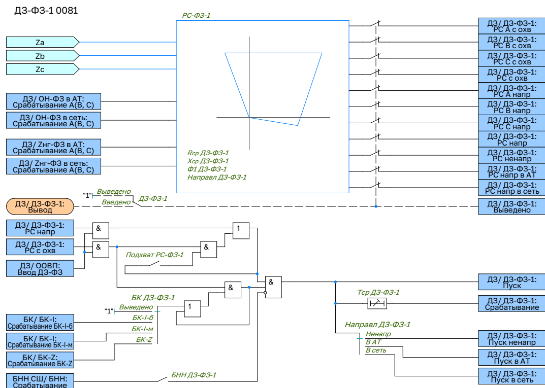
Рисунок 2.8 – Функциональная схема логики ДЗ-ФЗ-1
