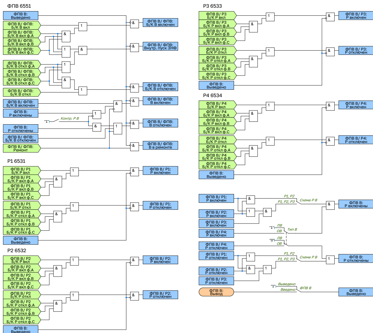
Рисунок 2.46 – Функциональная схема логики ФПВ В2
