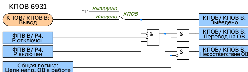
Рисунок 2.49 – Функциональная схема логики контроля перевода на ОВ
